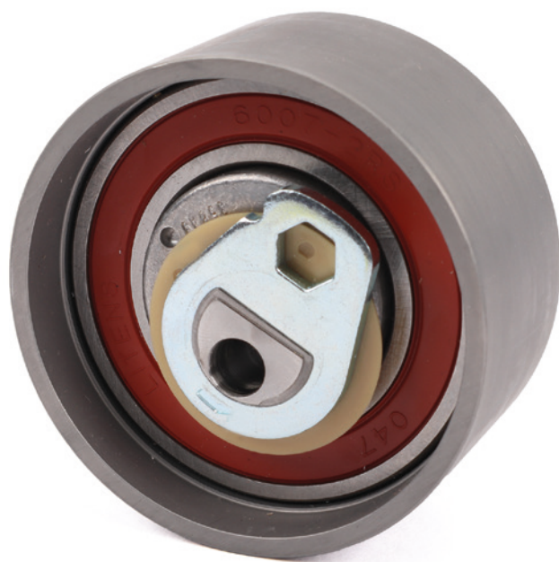
Εικόνα 2: Νέος σχεδιασμός με ατσάλινη επιφάνεια κύλισης
