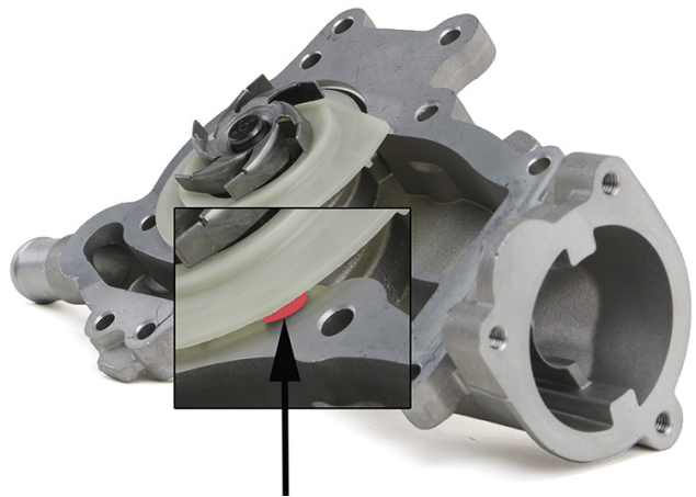
Εικόνα 2: Στρέβλωση πλαστικού προστατευτικού στοιχείου λόγω χρήσης κόλλας στεγανοποίησης
